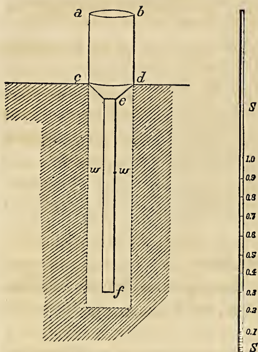
RAIN GAGE.
